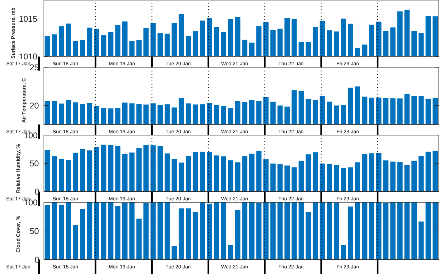
Met Forecast for CSA (ONHYM) PPL EBS - Senegal from 18-Jan-2026 00:00:00 to 25-Jan-2026 00:00:00
