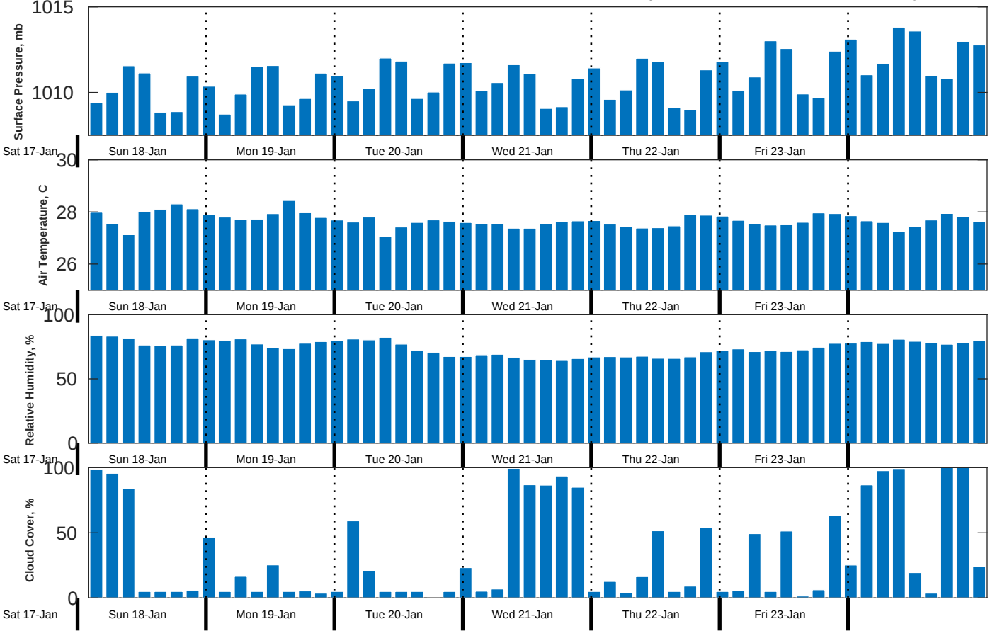
Met Forecast for CSA (ONHYM) PPL EBS - Sierra Leone from 18-Jan-2026 00:00:00 to 25-Jan-2026 00:00:00
