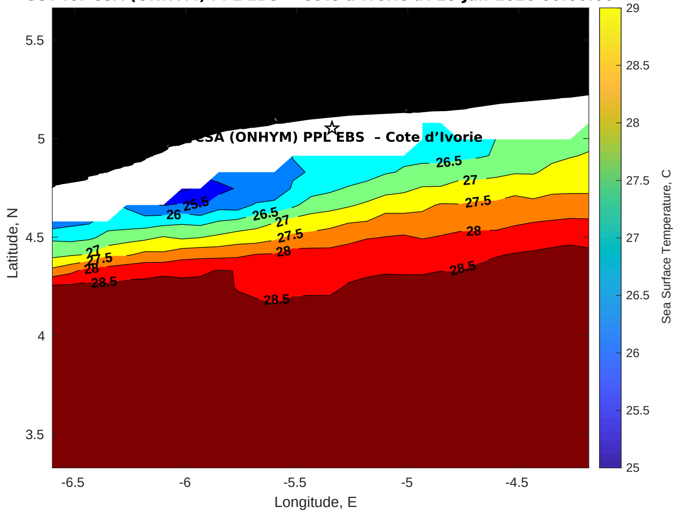
SST for CSA (ONHYM) PPL EBS - Cote d'Ivoire at 18-Jan-2026 00:00:00
