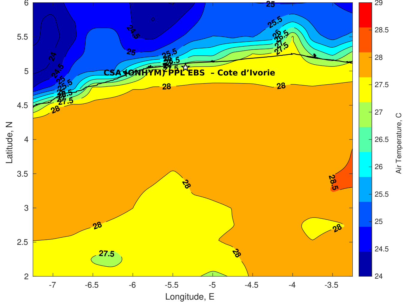
Air Temperature (C) for CSA (ONHYM) PPL EBS - Cote d'Ivoire at 19-Jan-2026
