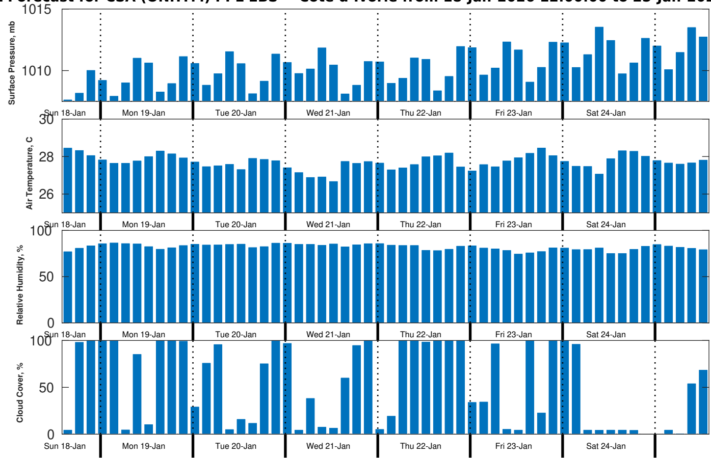
Met Forecast for CSA (ONHYM) PPL EBS - Cote d'Ivoire from 18-Jan-2026 12:00:00 to 25-Jan-2026 12:00:00
