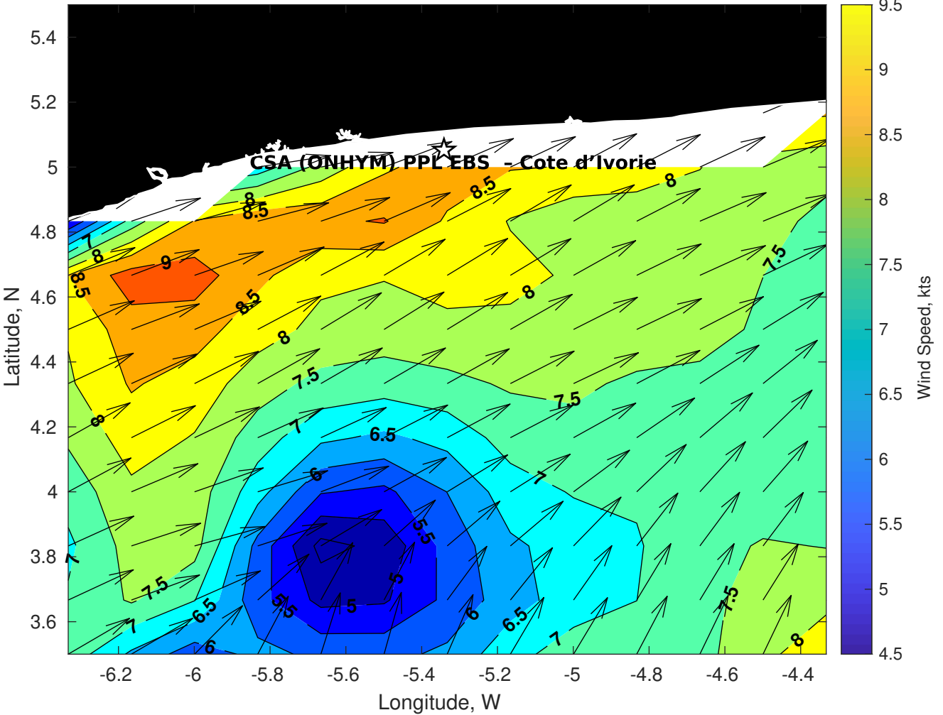
GFS Winds (kts) for CSA (ONHYM) PPL EBS - Cote d'Ivoire at 19-Jan-2026 09:00:00
