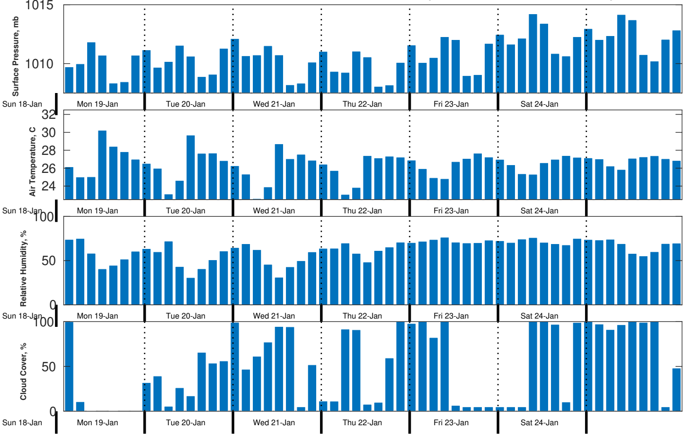
Met Forecast for CSA (ONHYM) PPL EBS - Guinea from 19-Jan-2026 00:00:00 to 26-Jan-2026 00:00:00
