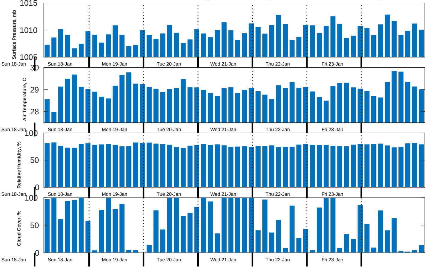
Met Forecast for CSA (ONHYM) PPL EBS - Nigeria from 19-Jan-2026 00:00:00 to 26-Jan-2026 00:00:00
