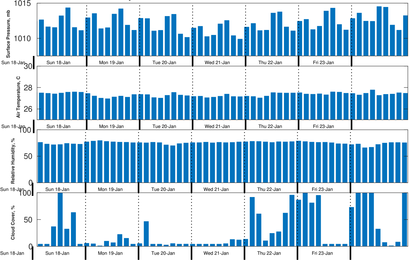
Met Forecast for Gyre from 18-Jan-2026 20:00:00 to 25-Jan-2026 20:00:00
