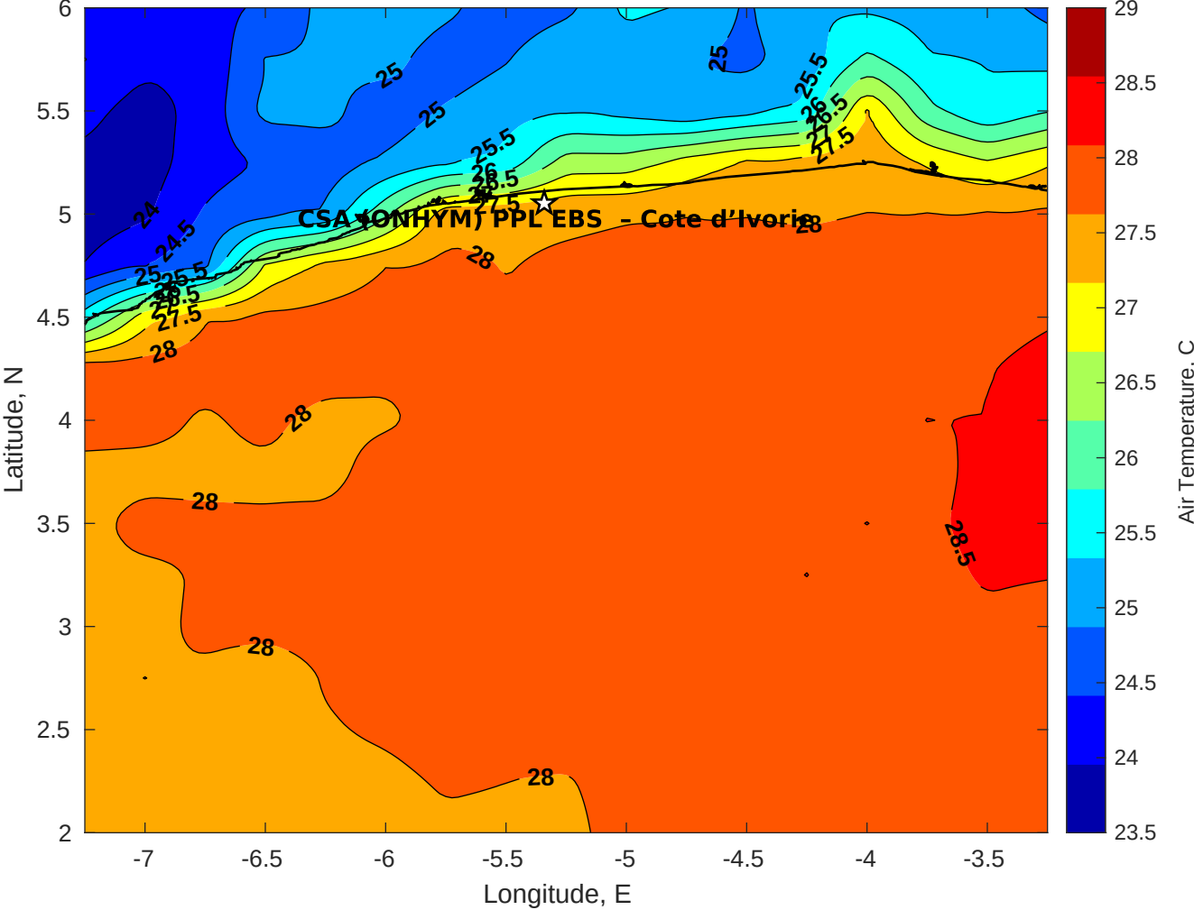
Air Temperature (C) for CSA (ONHYM) PPL EBS - Cote d'Ivoire at 20-Jan-2026
