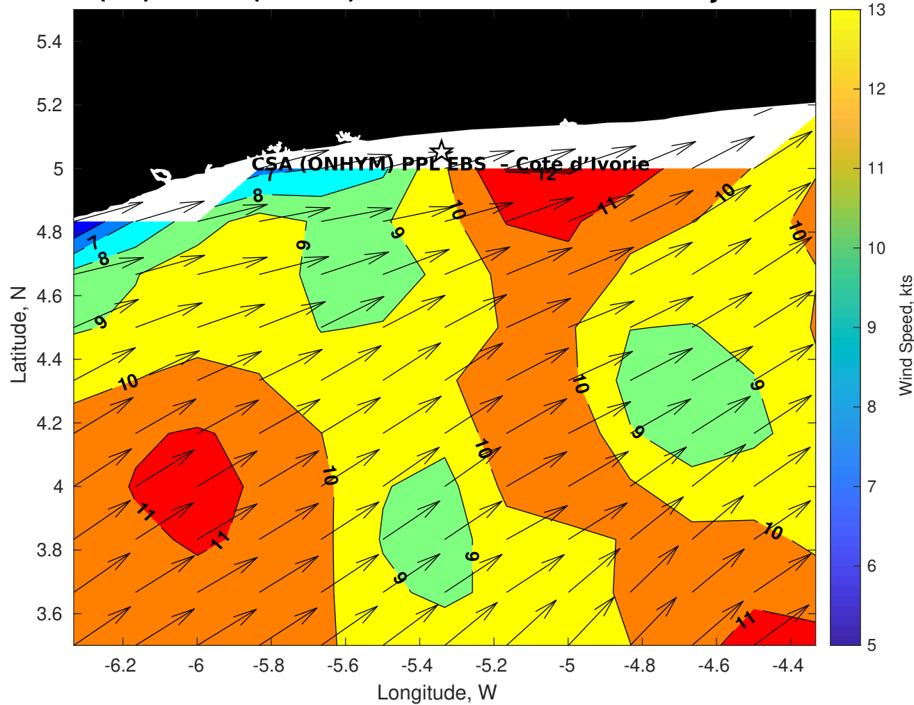
GFS Winds (kts) for CSA (ONHYM) PPL EBS - Cote d'Ivoire at 20-Jan-2026 09:00:00
