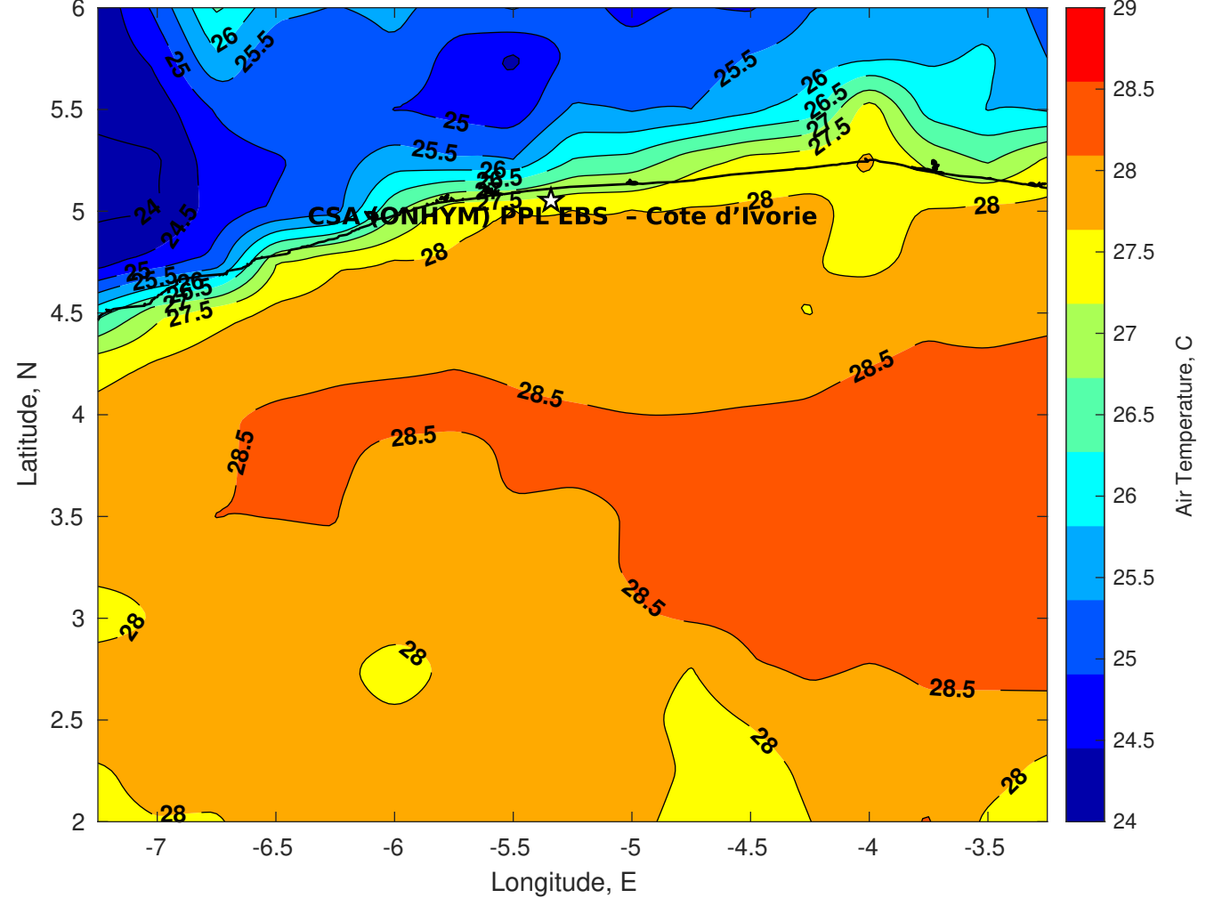
Air Temperature (C) for CSA (ONHYM) PPL EBS - Cote d'Ivoire at 20-Jan-2026
