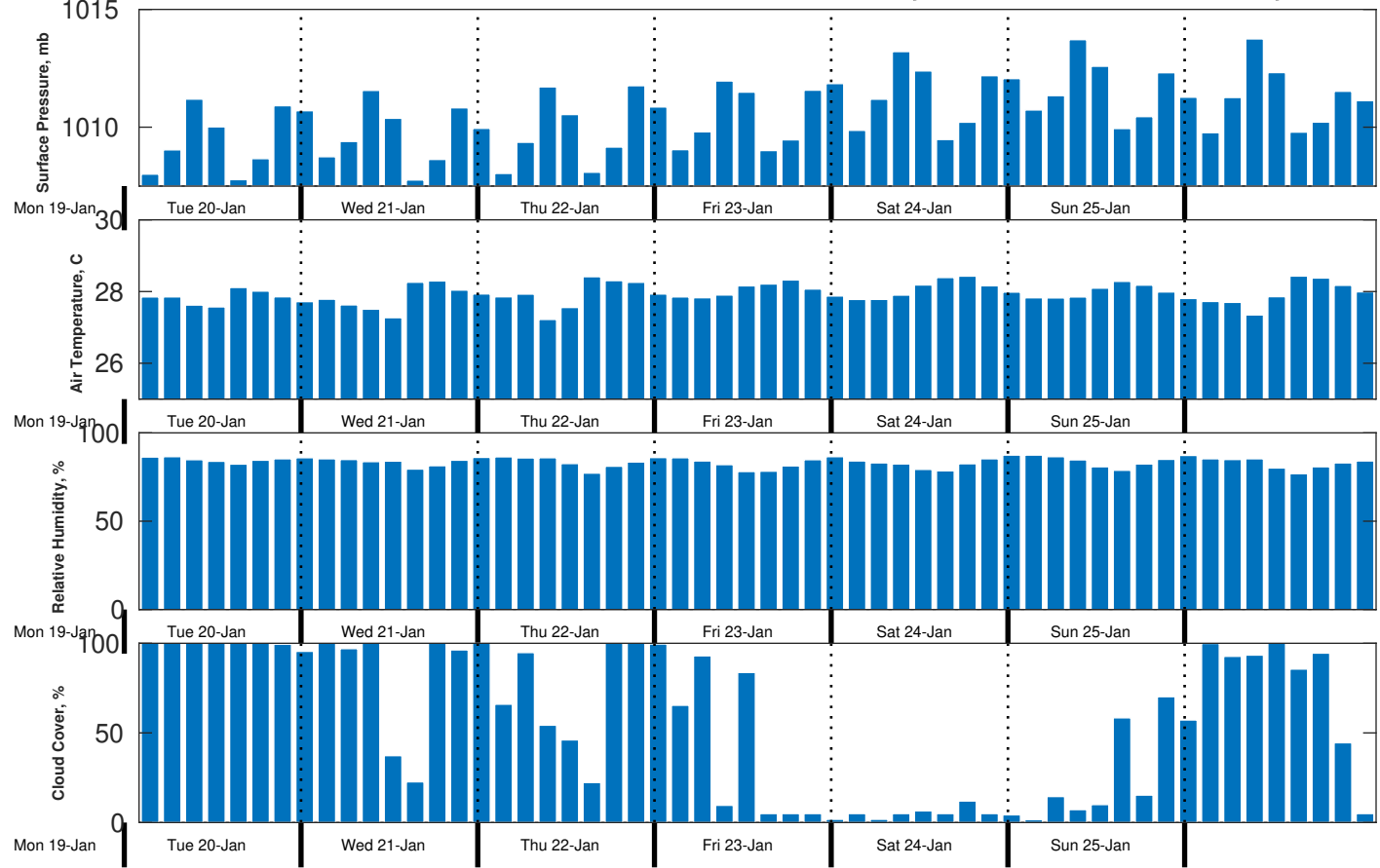
Met Forecast for CSA (ONHYM) PPL EBS - Cote d'Ivoire from 20-Jan-2026 00:00:00 to 27-Jan-2026 00:00:00
