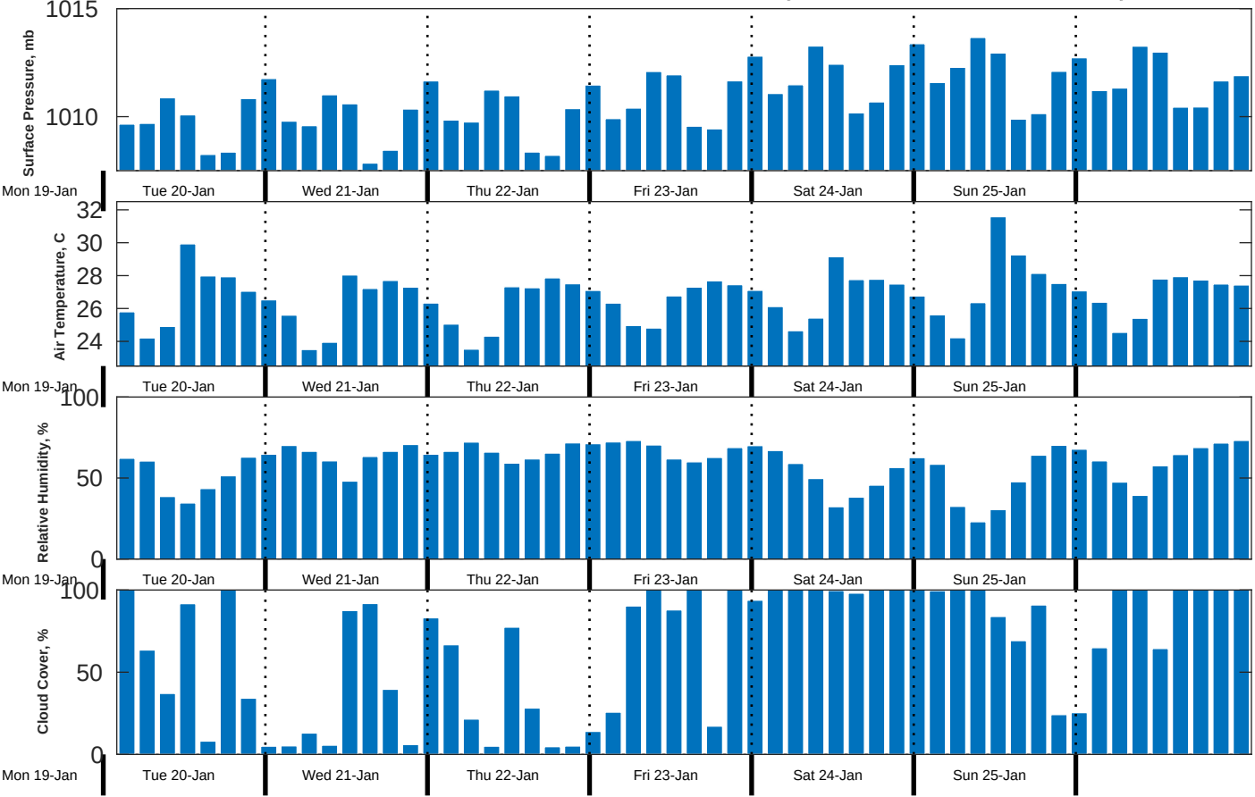
Met Forecast for CSA (ONHYM) PPL EBS - Guinea from 20-Jan-2026 00:00:00 to 27-Jan-2026 00:00:00
