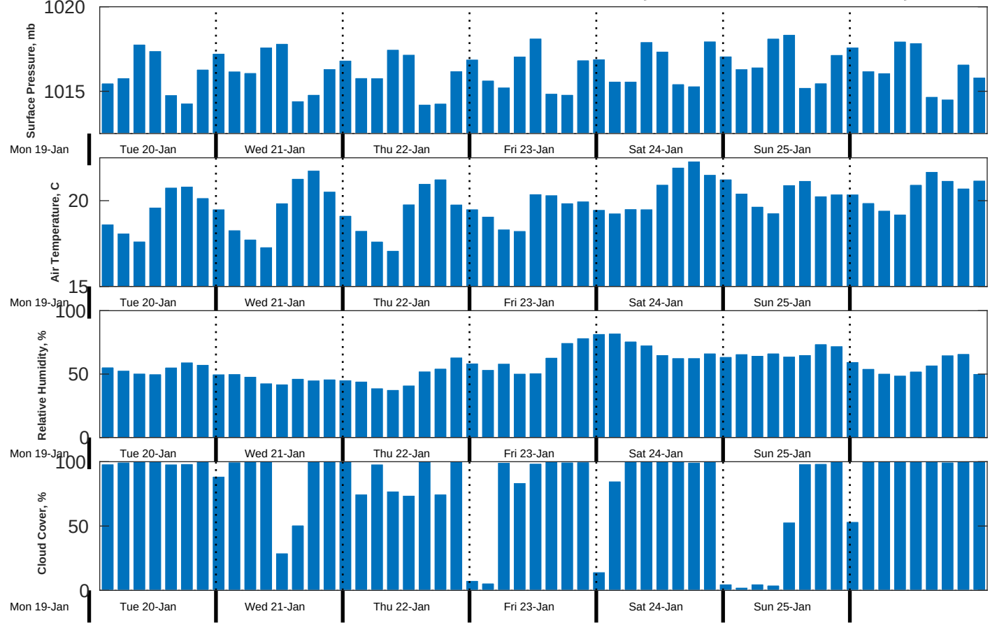
Met Forecast for CSA (ONHYM) PPL EBS - Mauritania from 20-Jan-2026 00:00:00 to 27-Jan-2026 00:00:00
