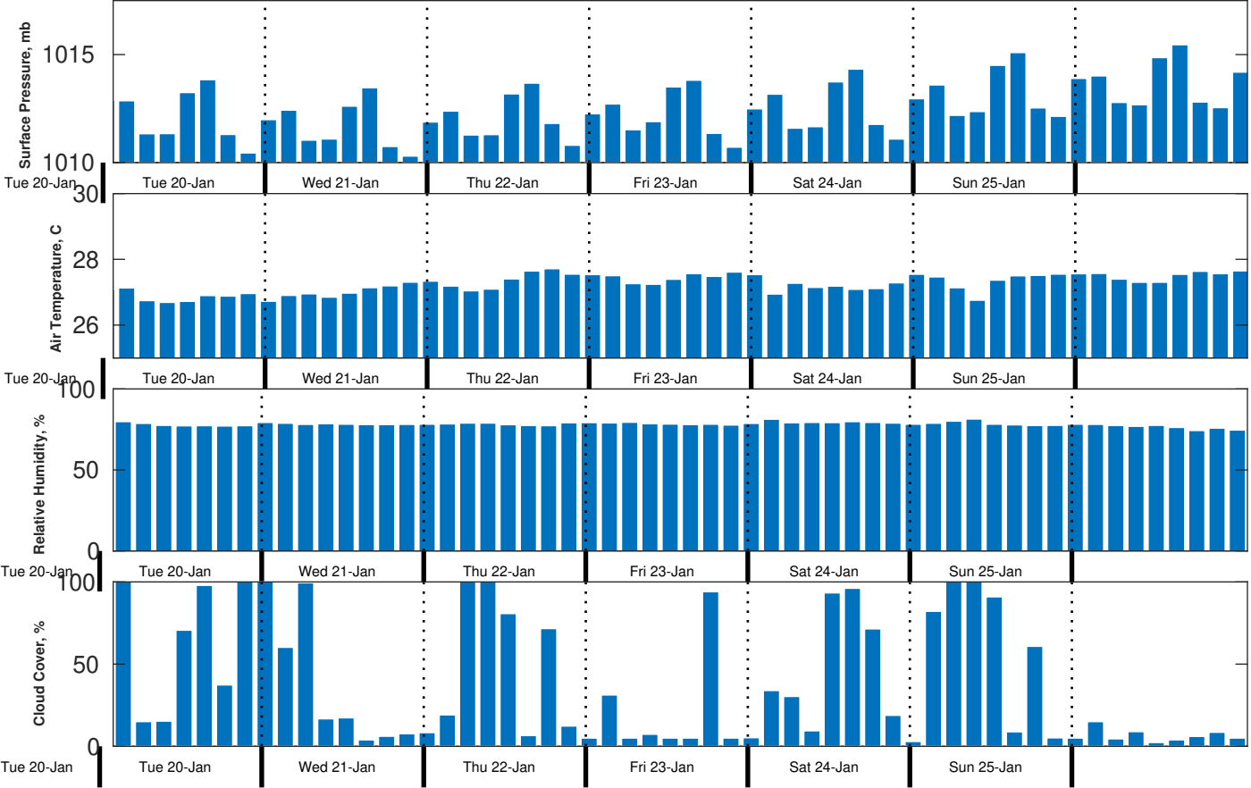
Met Forecast for Gyre from 20-Jan-2026 20:00:00 to 27-Jan-2026 20:00:00
