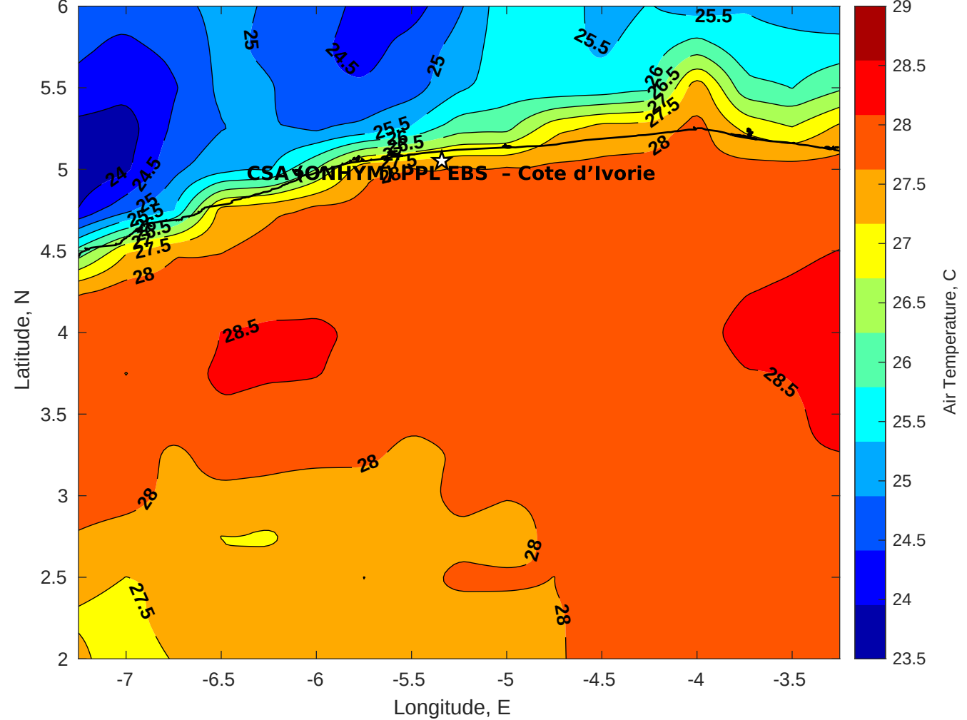
Air Temperature (C) for CSA (ONHYM) PPL EBS - Cote d'Ivoire at 22-Jan-2026
