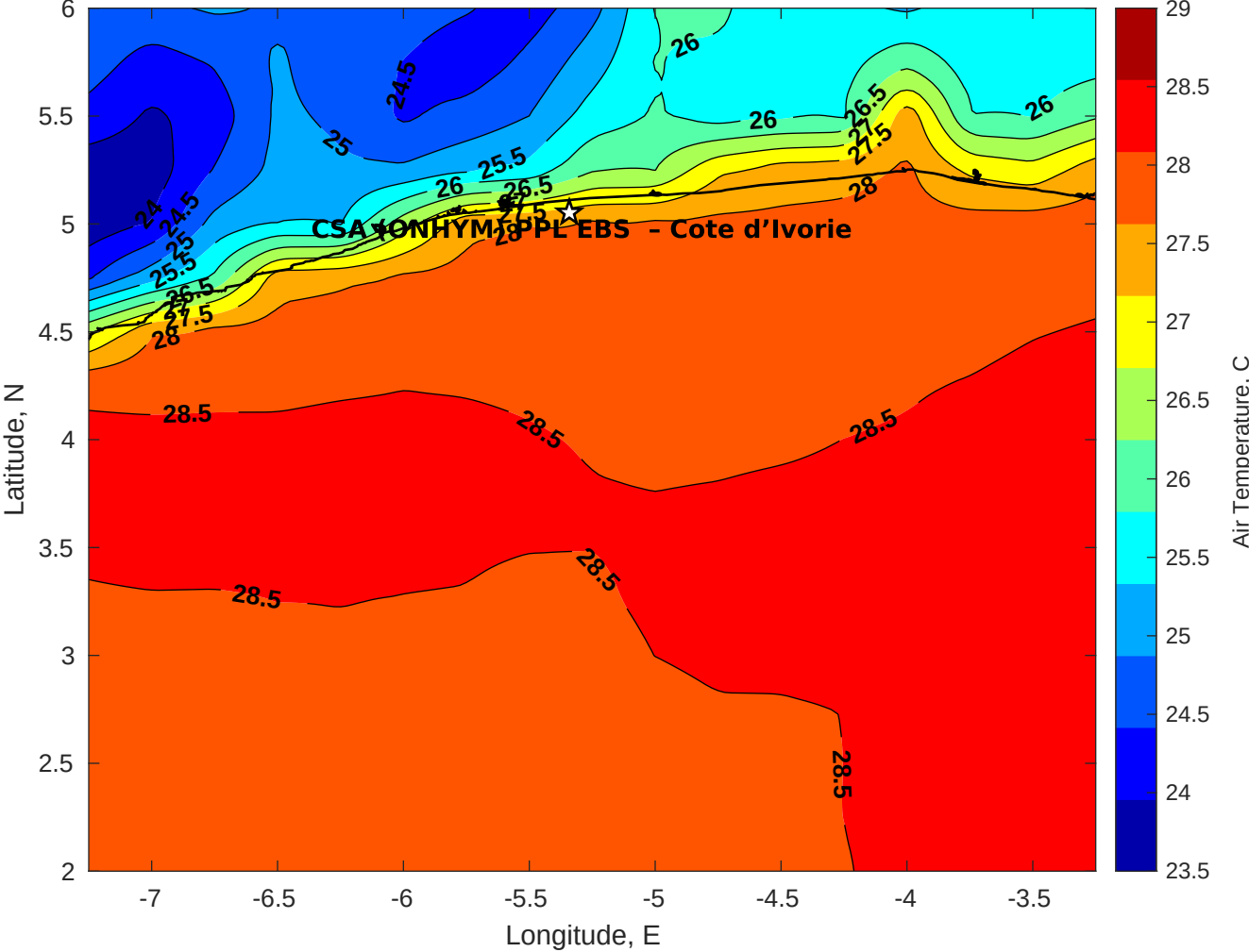
Air Temperature (C) for CSA (ONHYM) PPL EBS - Cote d'Ivoire at 22-Jan-2026
