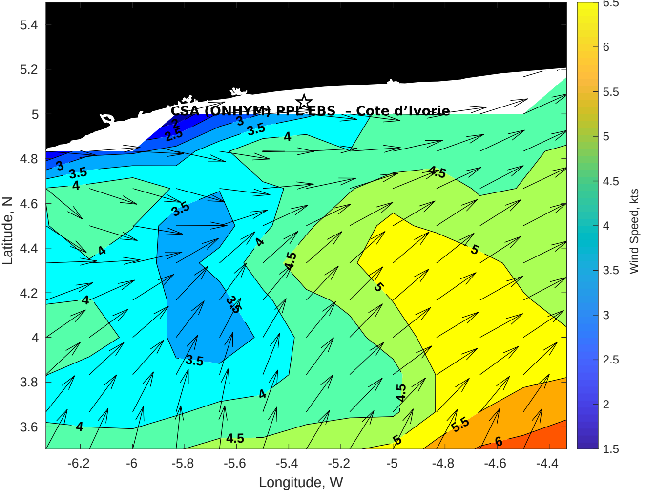
GFS Winds (kts) for CSA (ONHYM) PPL EBS - Cote d'Ivoire at 22-Jan-2026 09:00:00
