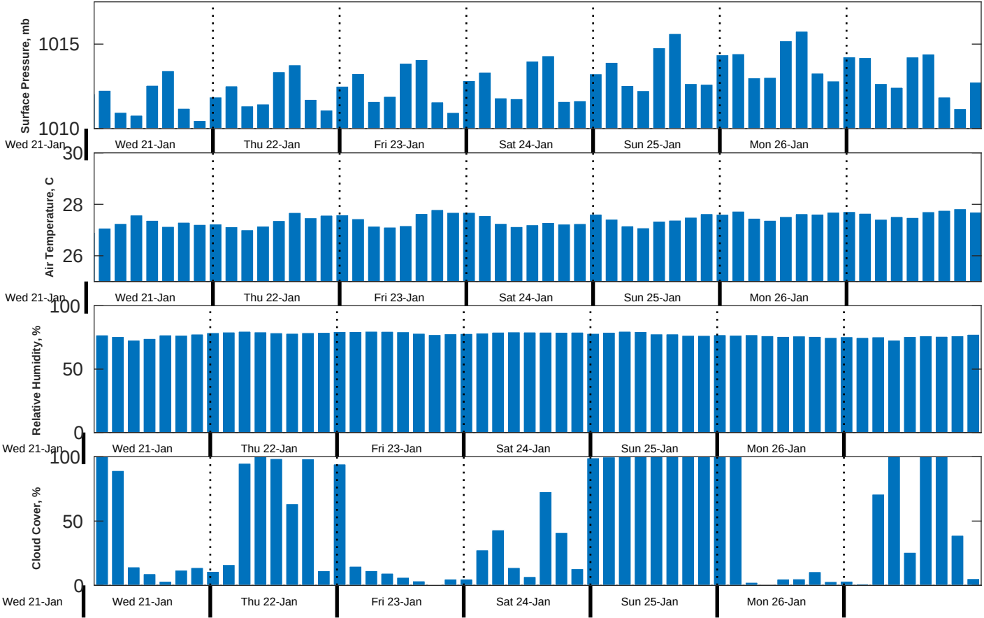
Met Forecast for Gyre from 21-Jan-2026 20:00:00 to 28-Jan-2026 20:00:00
