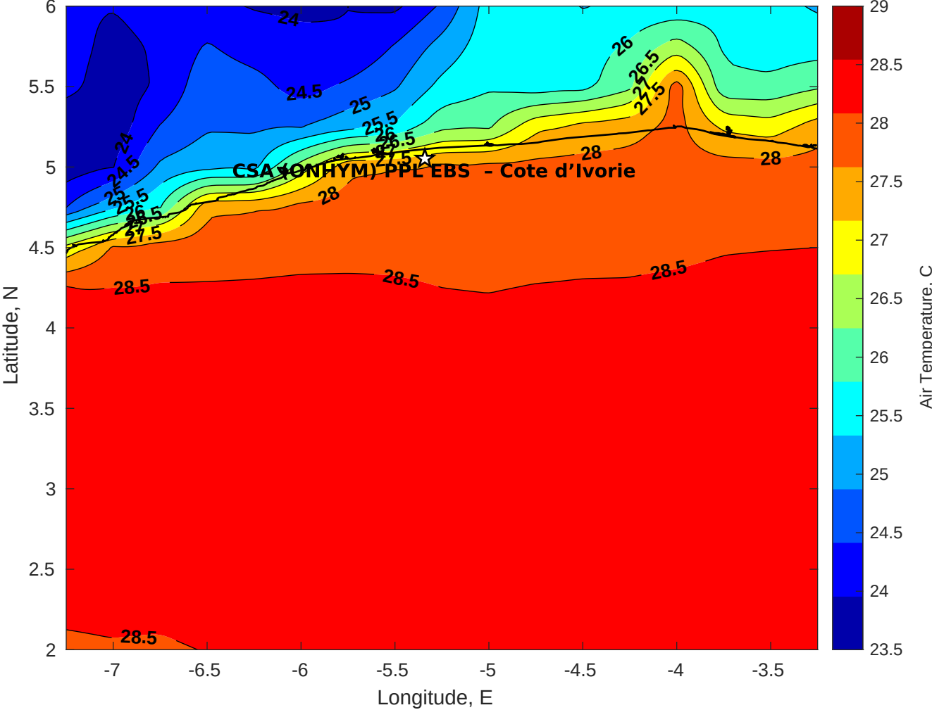
Air Temperature (C) for CSA (ONHYM) PPL EBS - Cote d'Ivoire at 23-Jan-2026
