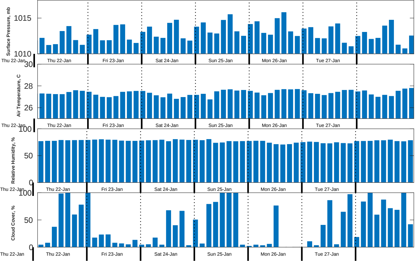
Met Forecast for Gyre from 22-Jan-2026 20:00:00 to 29-Jan-2026 20:00:00
