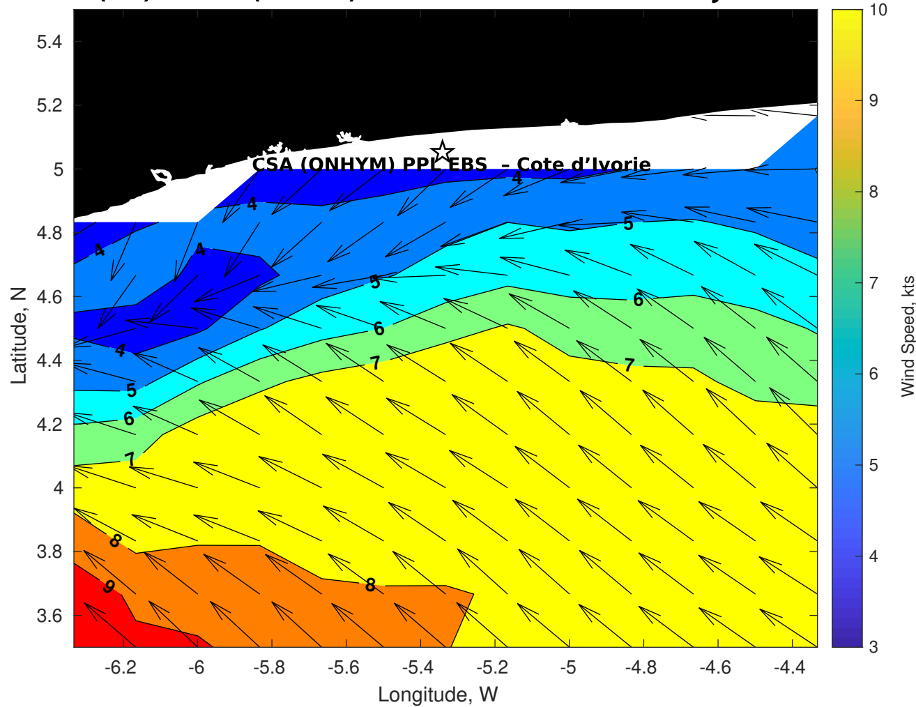
GFS Winds (kts) for CSA (ONHYM) PPL EBS - Cote d'Ivoire at 24-Jan-2026 09:00:00
