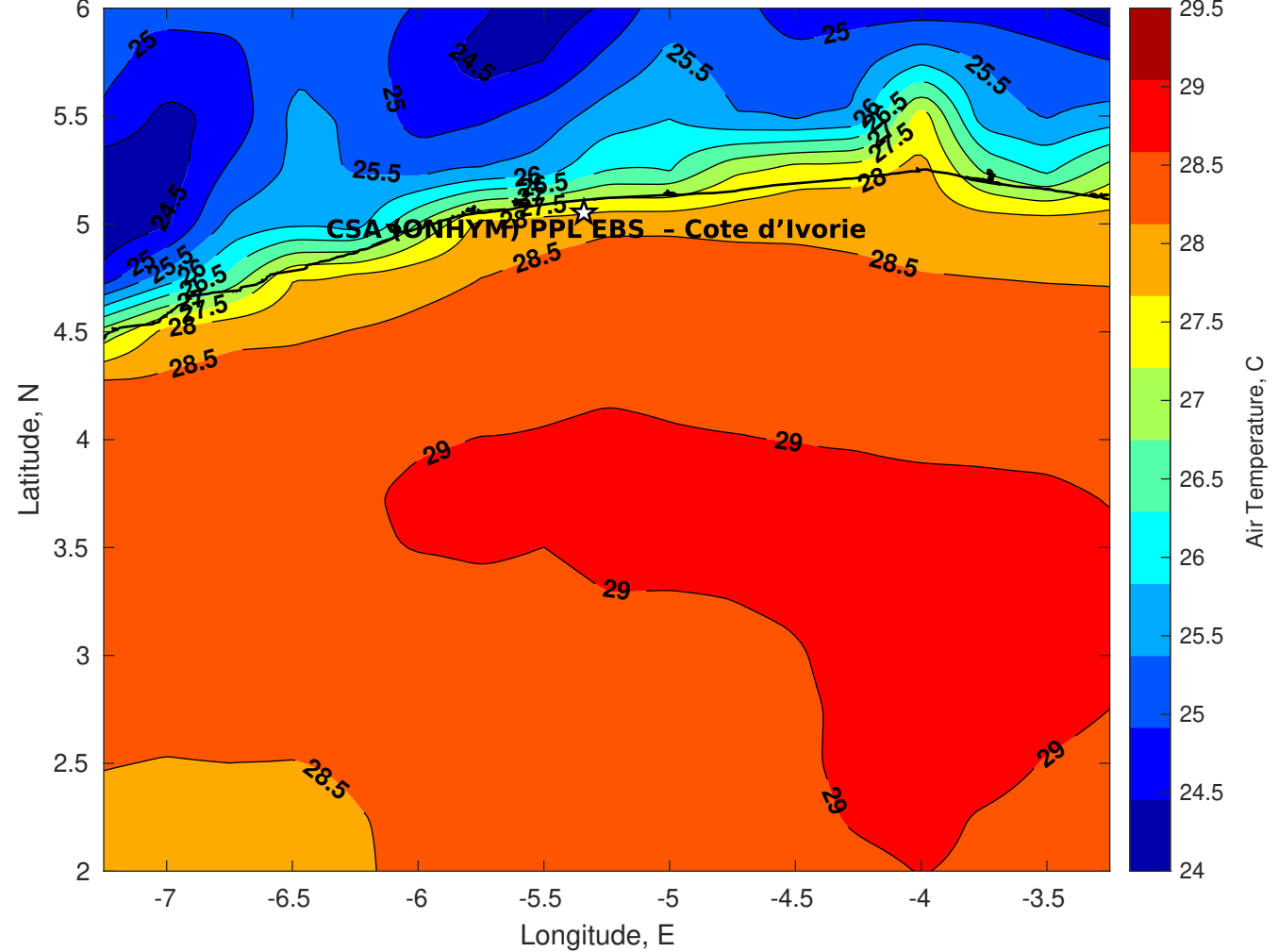
Air Temperature (C) for CSA (ONHYM) PPL EBS - Cote d'Ivoire at 24-Jan-2026
