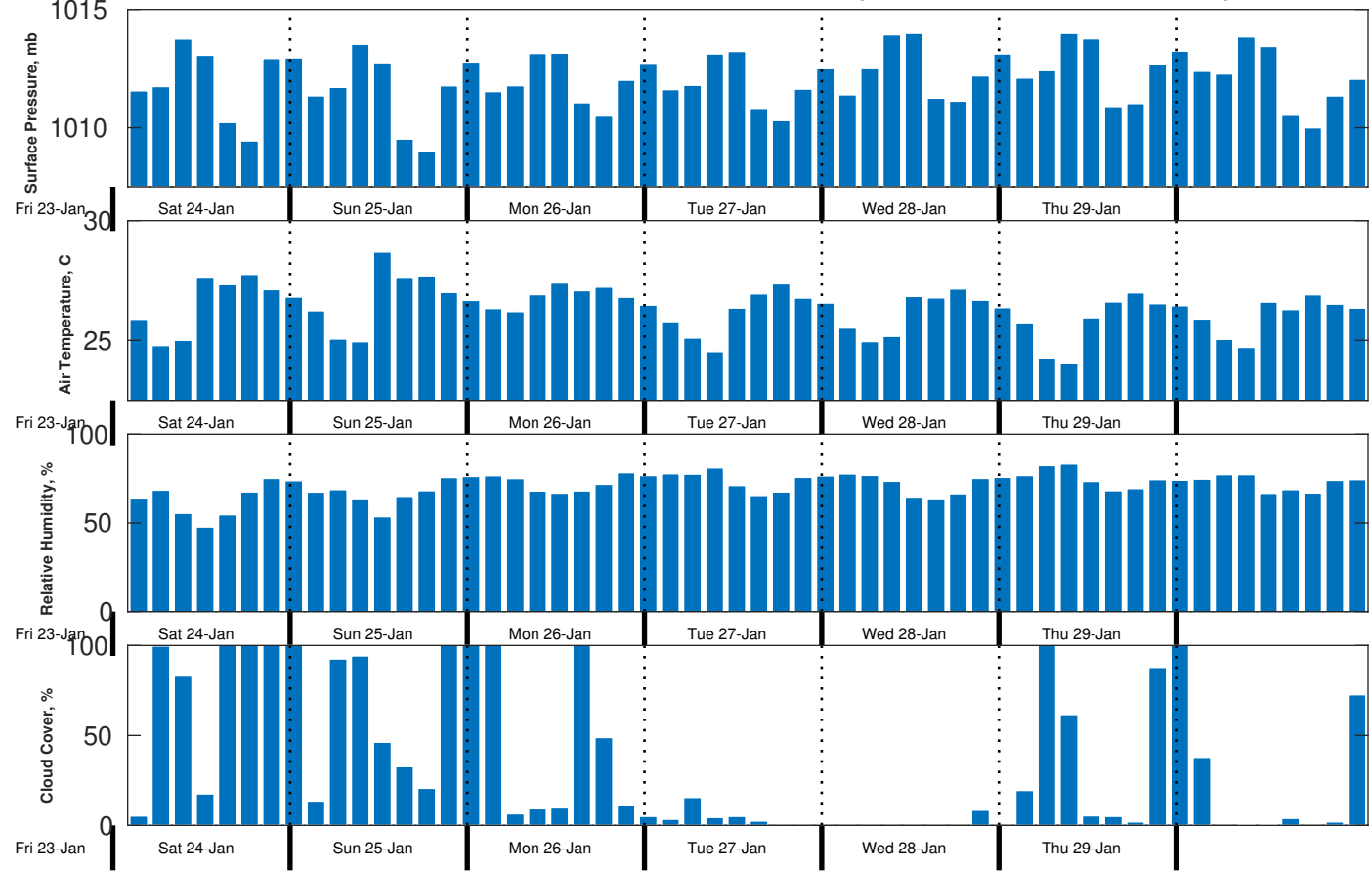
Met Forecast for CSA (ONHYM) PPL EBS - Guinea from 24-Jan-2026 00:00:00 to 31-Jan-2026 00:00:00
