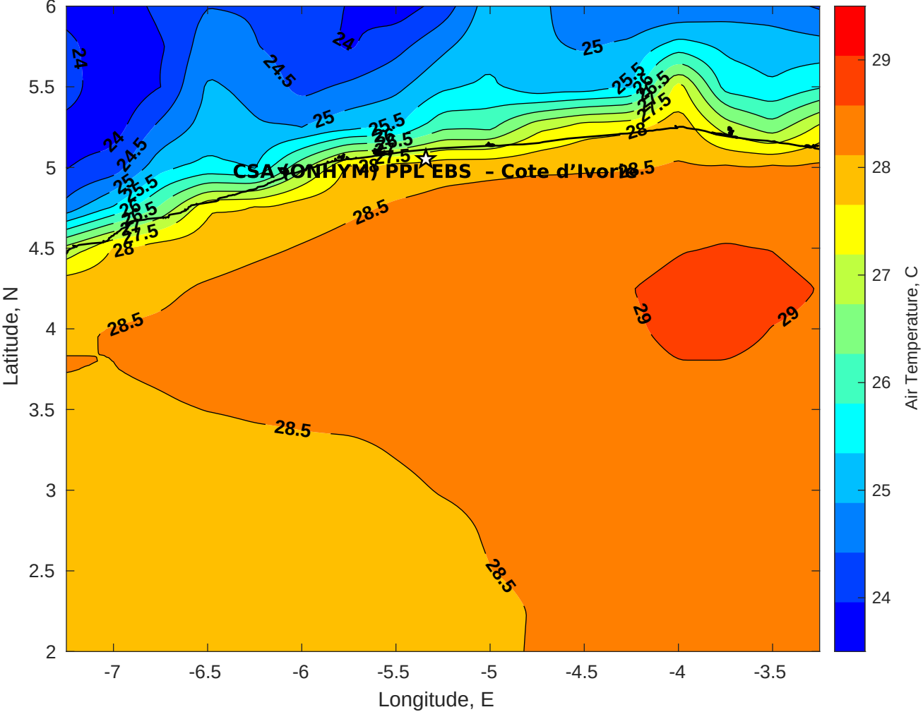
Air Temperature (C) for CSA (ONHYM) PPL EBS - Cote d'Ivoire at 25-Jan-2026
