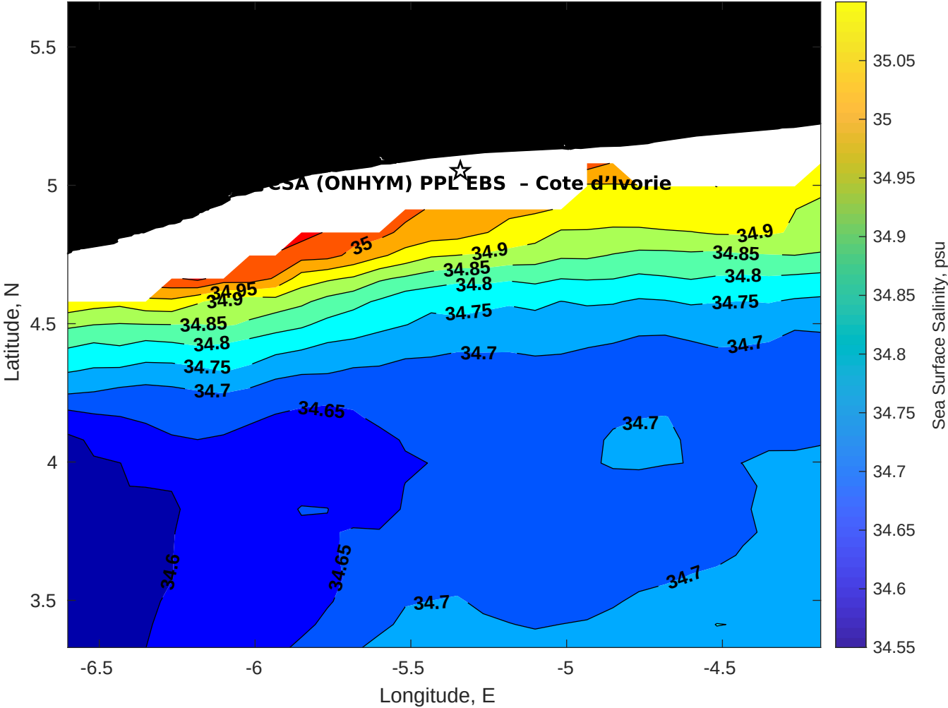
Surface Salinity for CSA (ONHYM) PPL EBS - Cote d'Ivoire at 24-Jan-2026 00:00:00
