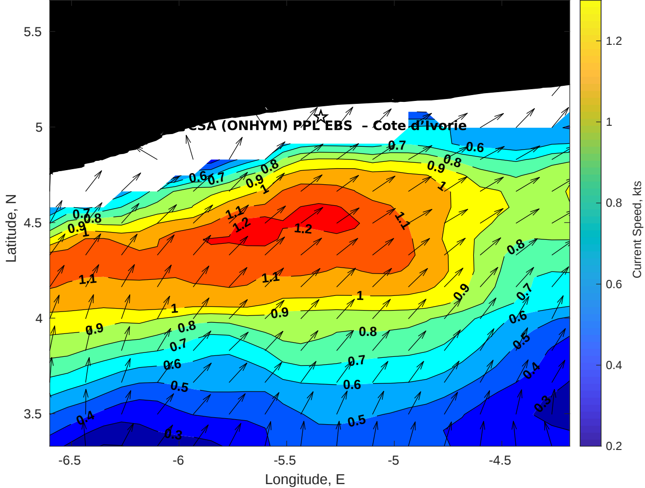
Surface Currents for CSA (ONHYM) PPL EBS - Cote d'Ivoire at 25-Jan-2026 00:00:00
