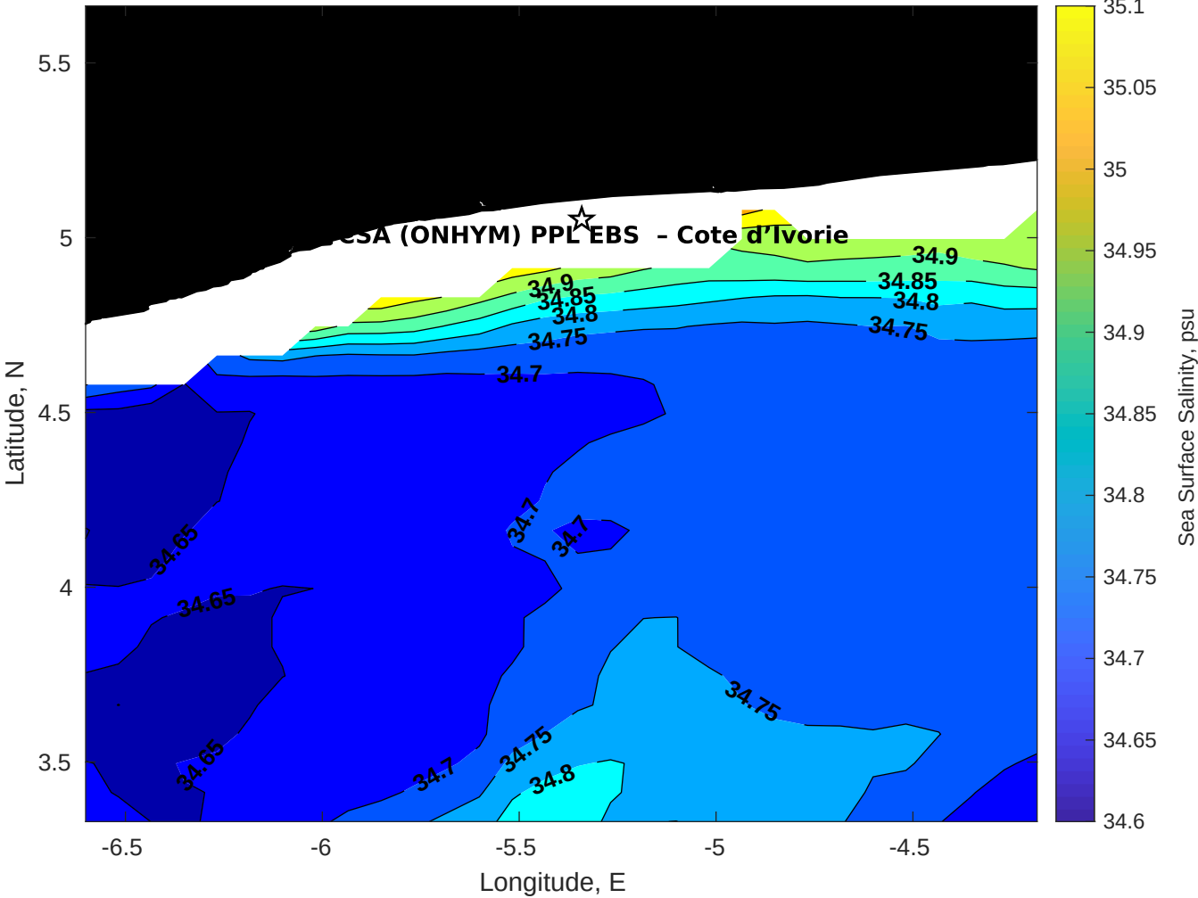
Surface Salinity for CSA (ONHYM) PPL EBS - Cote d'Ivoire at 26-Jan-2026 00:00:00
