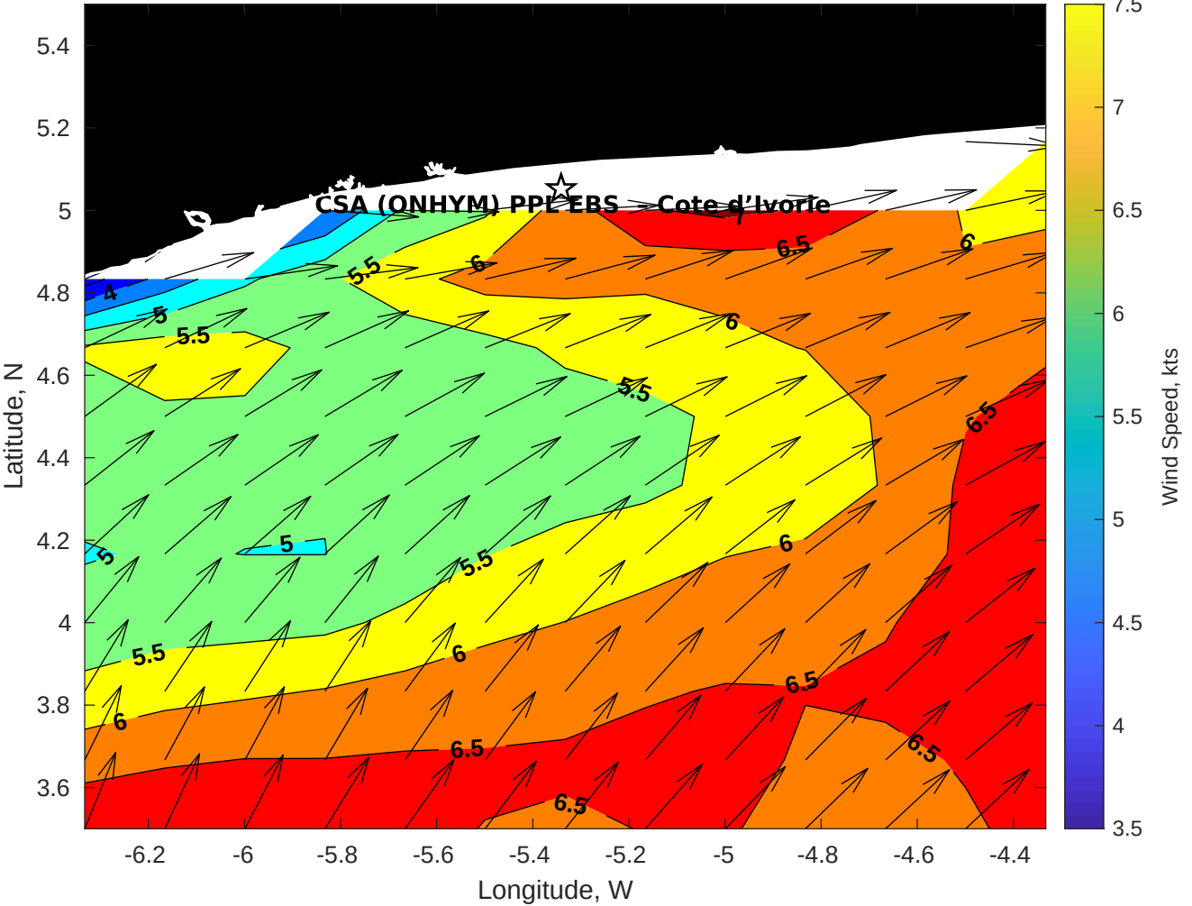
GFS Winds (kts) for CSA (ONHYM) PPL EBS - Cote d'Ivoire at 27-Jan-2026 09:00:00
