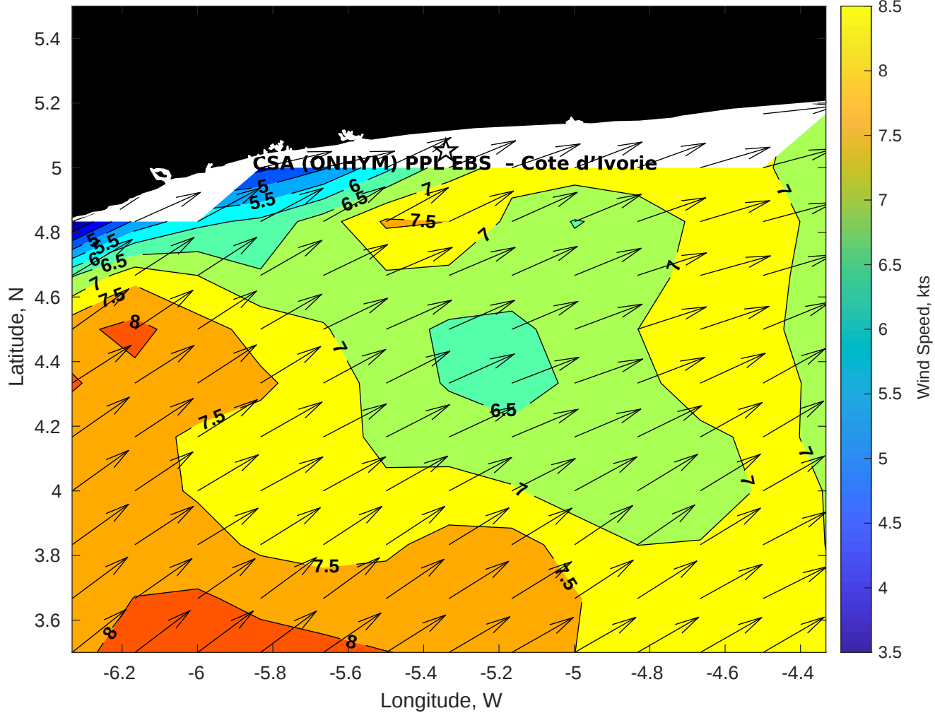
GFS Winds (kts) for CSA (ONHYM) PPL EBS - Cote d'Ivoire at 28-Jan-2026 09:00:00
