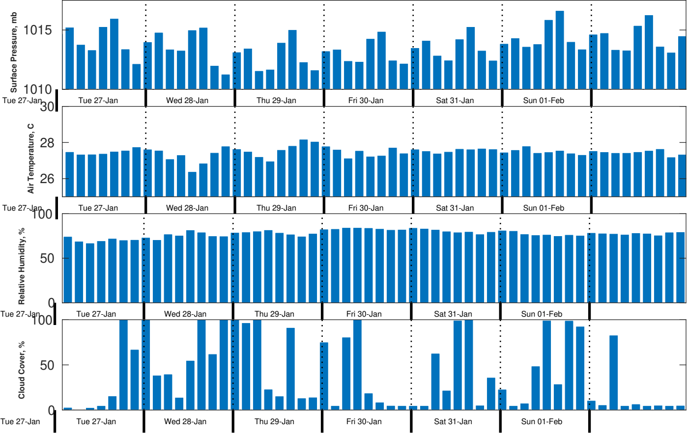
Met Forecast for Gyre from 27-Jan-2026 20:00:00 to 03-Feb-2026 20:00:00
