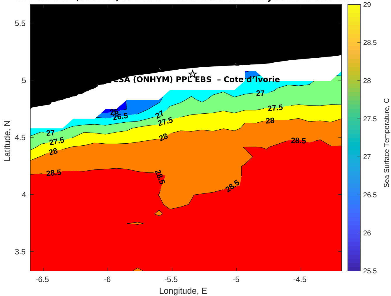
SST for CSA (ONHYM) PPL EBS - Cote d'Ivoire at 28-Jan-2026 00:00:00
