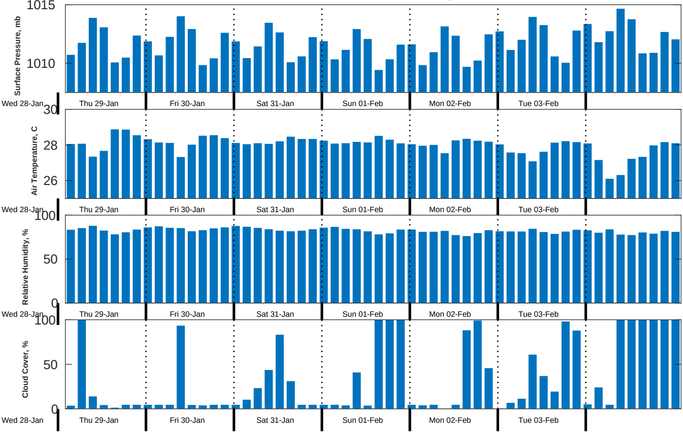
Met Forecast for CSA (ONHYM) PPL EBS - Cote d'Ivoire from 29-Jan-2026 00:00:00 to 05-Feb-2026 00:00:00
