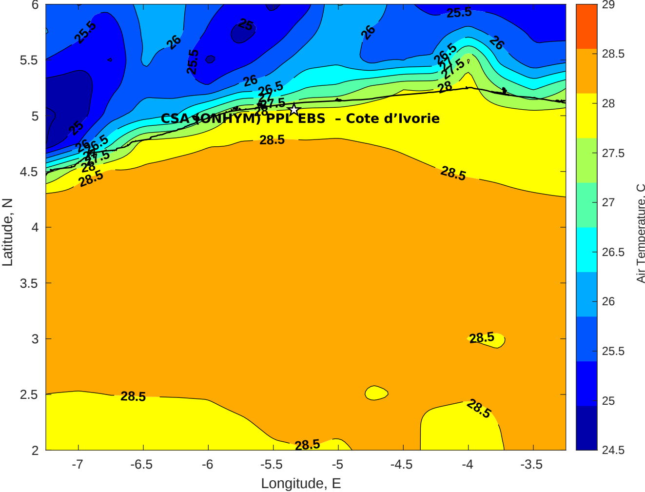
Air Temperature (C) for CSA (ONHYM) PPL EBS - Cote d'Ivoire at 30-Jan-2026
