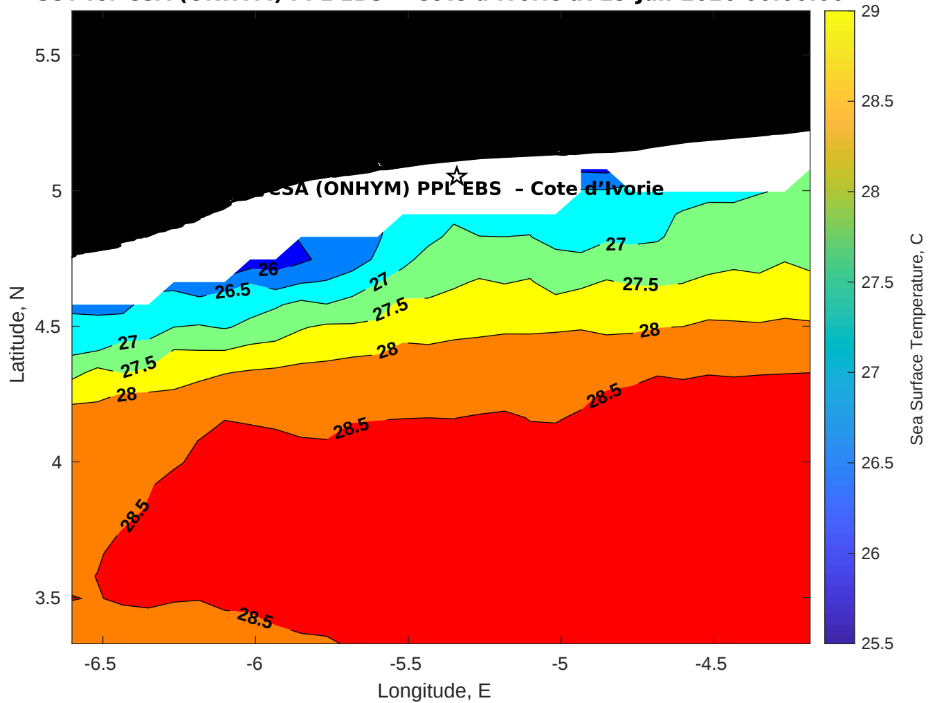
SST for CSA (ONHYM) PPL EBS - Cote d'Ivoire at 29-Jan-2026 00:00:00
