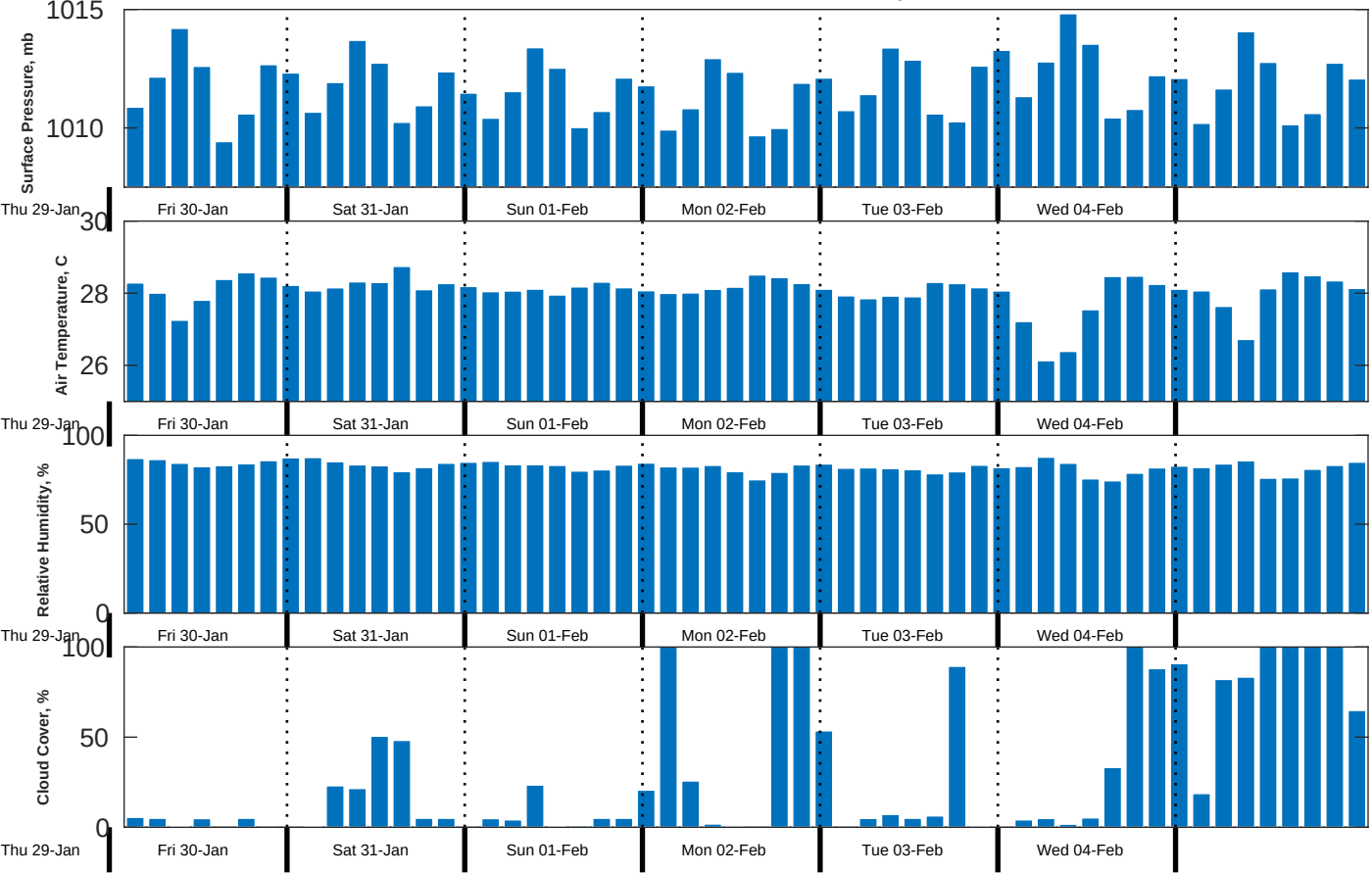
Met Forecast for CSA (ONHYM) PPL EBS - Cote d'Ivoire from 30-Jan-2026 00:00:00 to 06-Feb-2026 00:00:00
