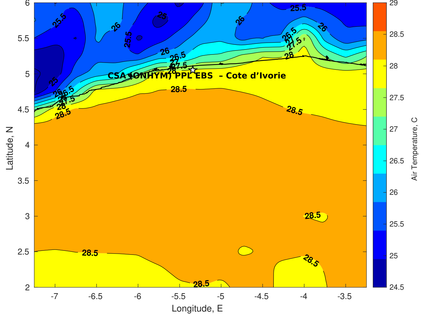
Air Temperature (C) for CSA (ONHYM) PPL EBS - Cote d'Ivoire at 30-Jan-2026
