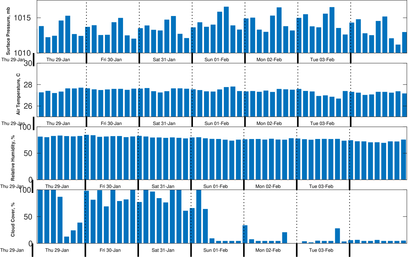
Met Forecast for Gyre from 29-Jan-2026 20:00:00 to 05-Feb-2026 20:00:00
