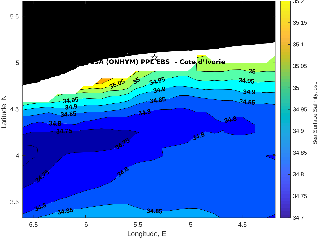
Surface Salinity for CSA (ONHYM) PPL EBS - Cote d'Ivoire at 30-Jan-2026 00:00:00
