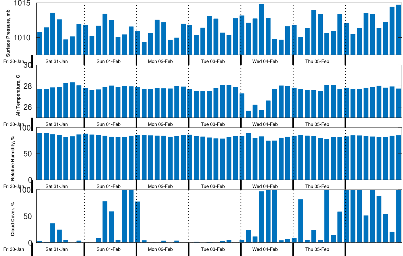
Met Forecast for CSA (ONHYM) PPL EBS - Cote d'Ivoire from 31-Jan-2026 00:00:00 to 07-Feb-2026 00:00:00
