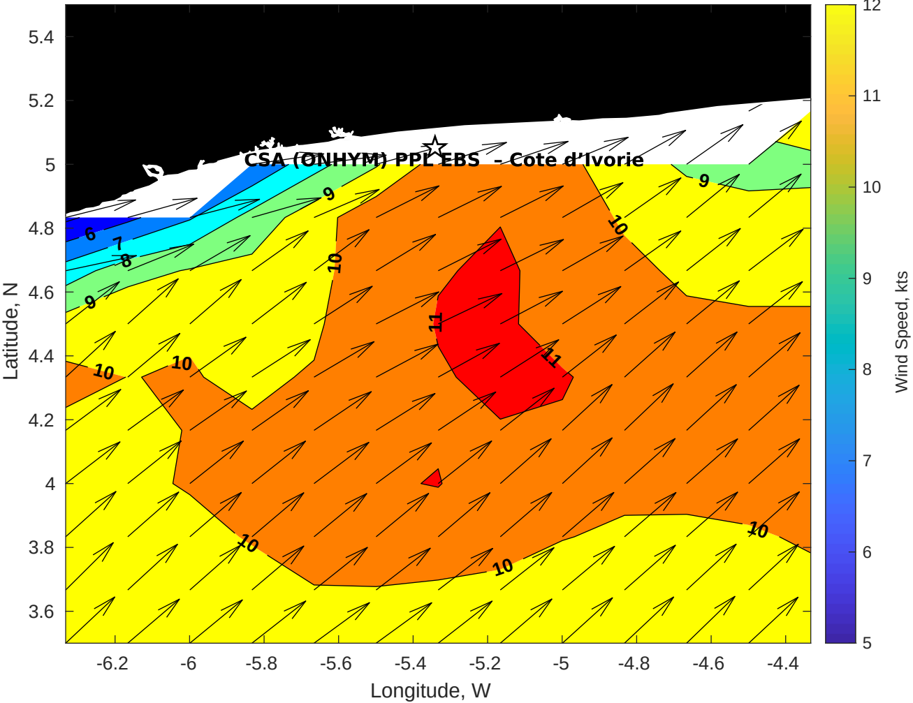
GFS Winds (kts) for CSA (ONHYM) PPL EBS - Cote d'Ivoire at 01-Feb-2026 09:00:00
