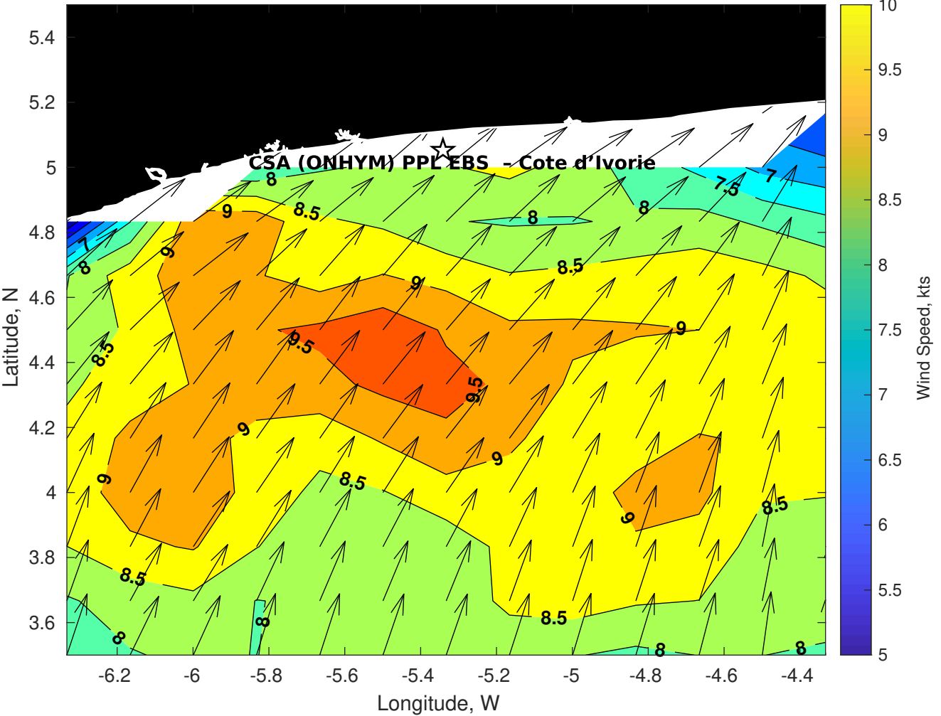
GFS Winds (kts) for CSA (ONHYM) PPL EBS - Cote d'Ivoire at 02-Feb-2026 09:00:00
