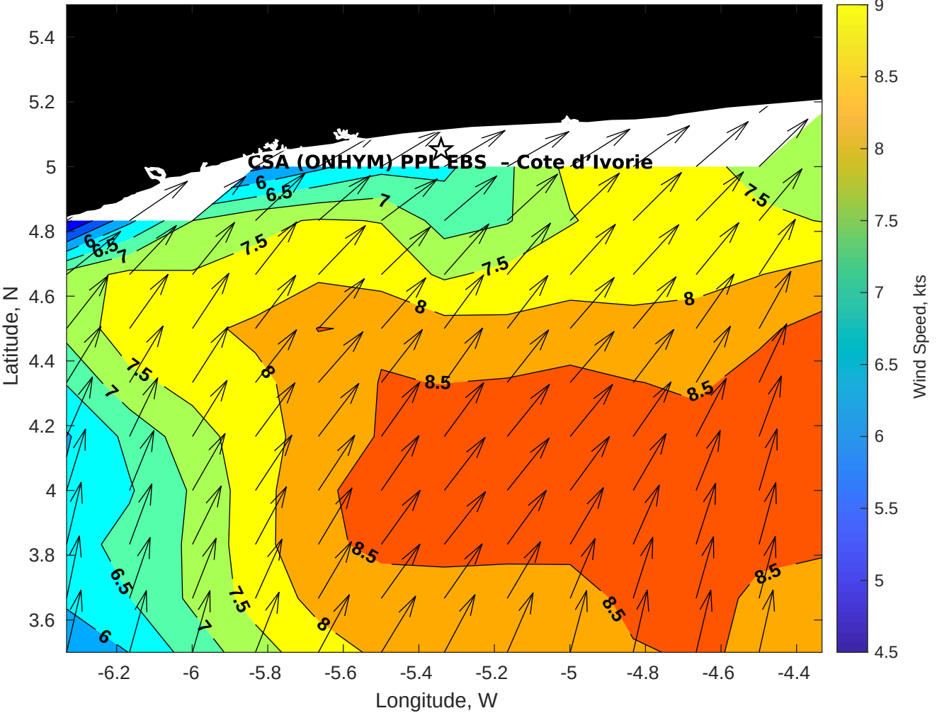
GFS Winds (kts) for CSA (ONHYM) PPL EBS - Cote d'Ivoire at 03-Feb-2026 09:00:00
