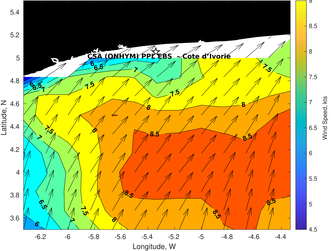
GFS Winds (kts) for CSA (ONHYM) PPL EBS - Cote d'Ivoire at 03-Feb-2026 09:00:00
