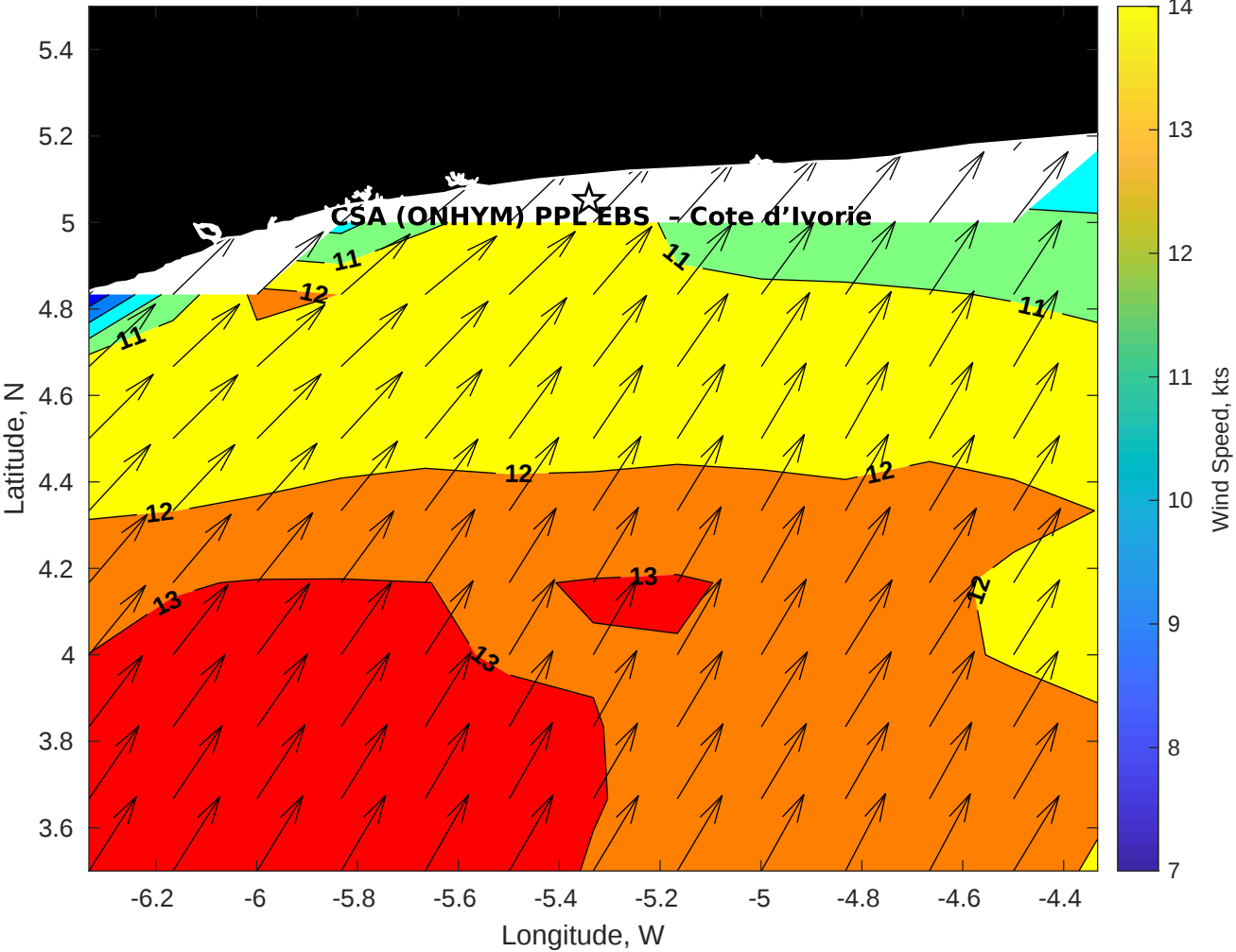
GFS Winds (kts) for CSA (ONHYM) PPL EBS - Cote d'Ivoire at 06-Feb-2026 09:00:00
