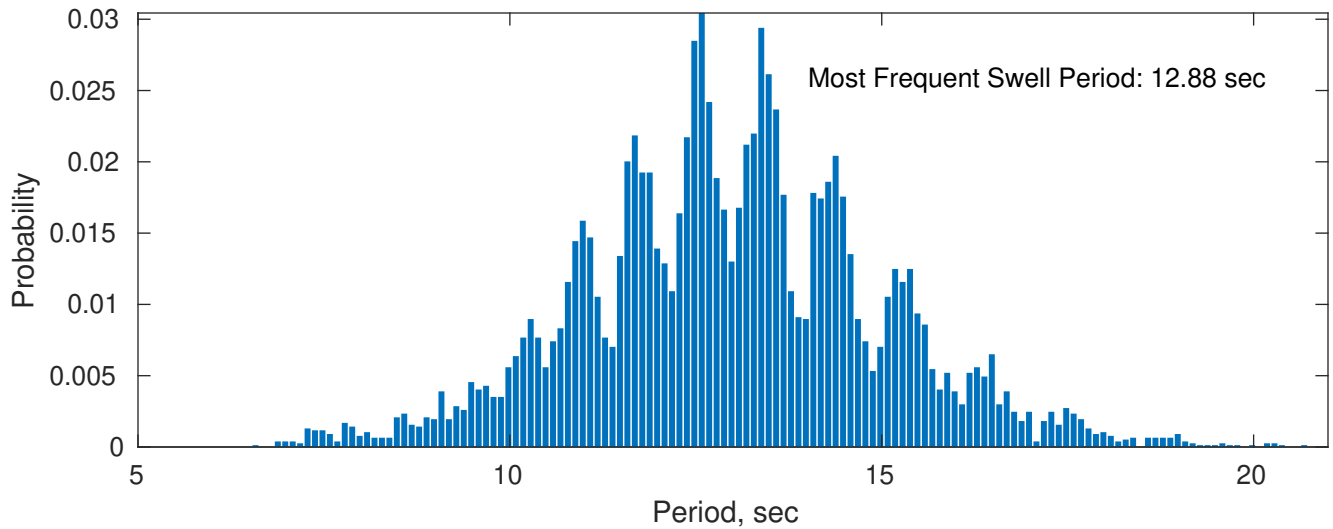
Swell: 96.46%
