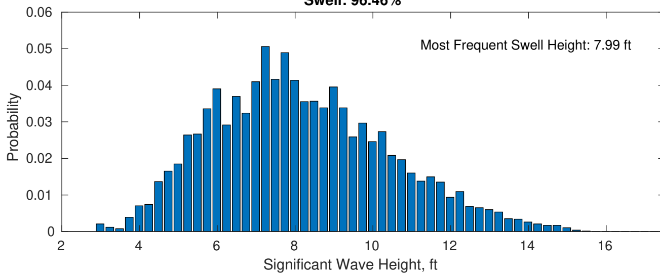
Swell: 96.46%
