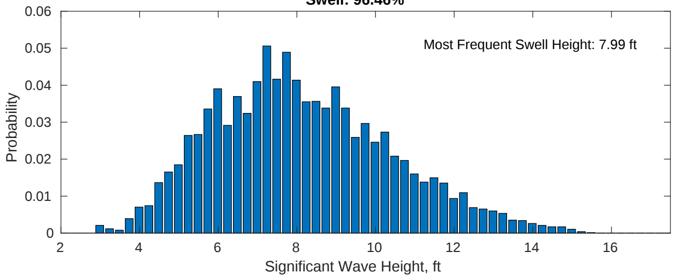
Swell: 96.46%
