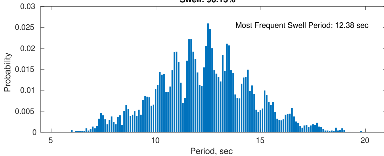
Swell: 96.13%
