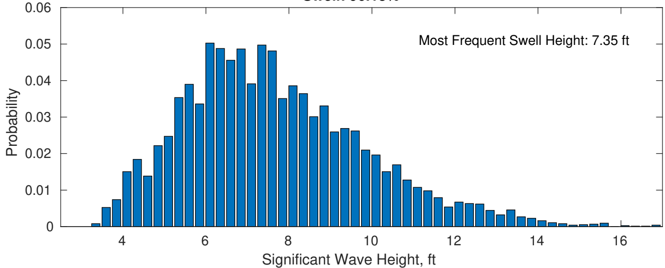
Swell: 96.13%
