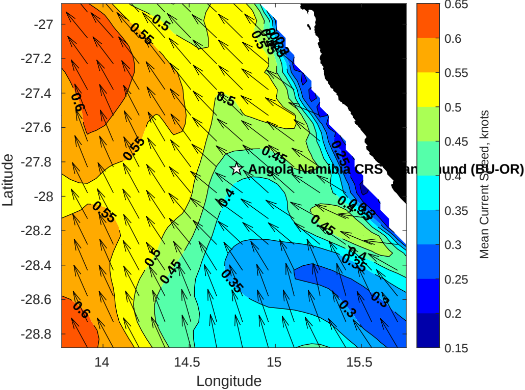
Angola Namibia CRS Oranjemund (BU-OR): May
