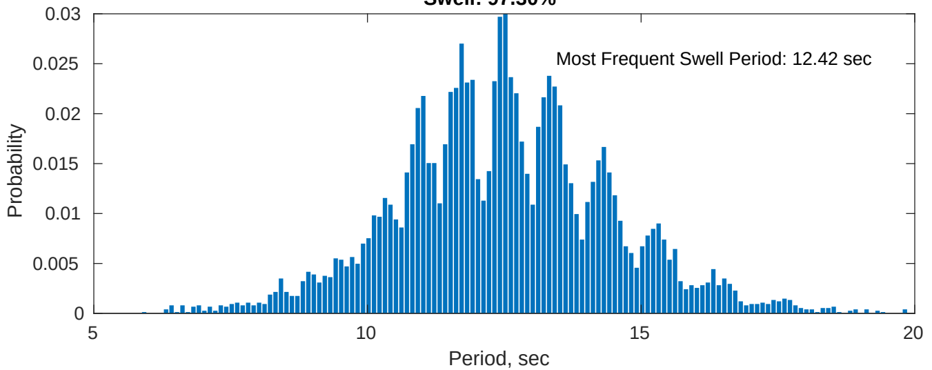
Swell: 97.30%
