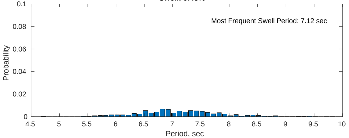
Swell: 9.43%
