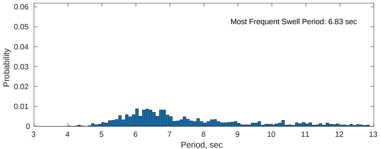
Swell: 21.83%
