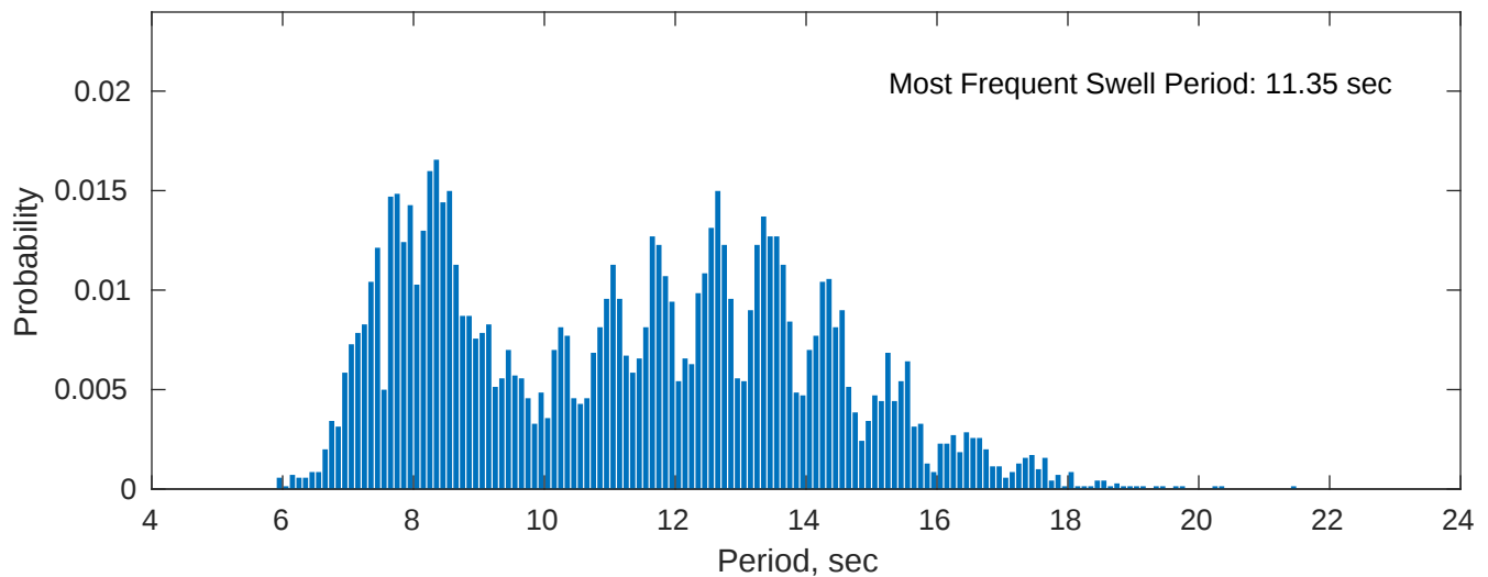
Swell: 79.59%
