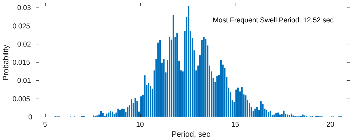
Swell: 90.56%
